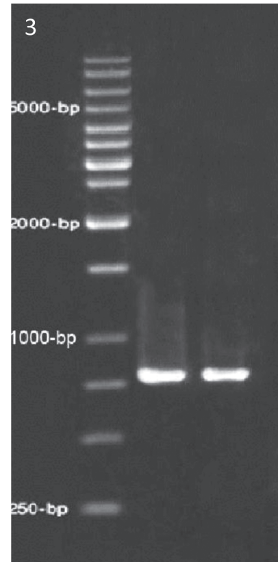
شکل ۱ الکتروفورز محصول PCR بر روی ژل آگاروز یک درصد ستون ۱ مارکر وزن مولکولی، ستون ۲ و ۳: قطعات تکثیر شده ژن LipL32 با پرایمرهای اختصاصی (۷۷۸ جفت باز)
