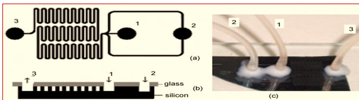
شکل ۴- الف) شماتیک، ب) سطح مقطع عرضی و ج) تصویر تراشه میکرو فلوئید ساخته شده توسط چن و همکاران، (۱) ورودی، (۲) ورودی بافر و (۳) خروجی دستگاه (۳۶)
