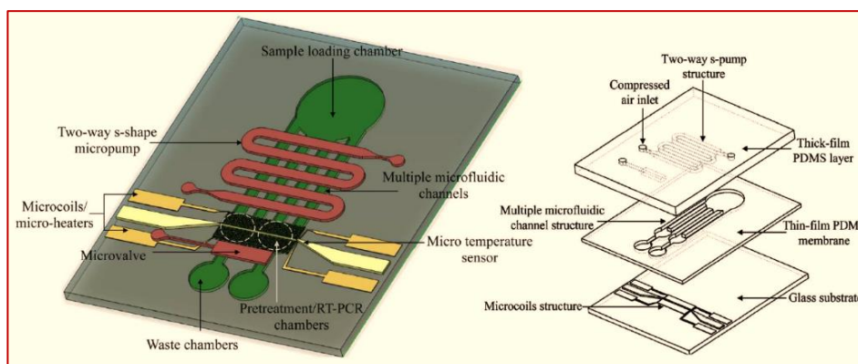
شکل ۱- شماتیک کلی تراشه‌ی RT-PCR (۳۲)
