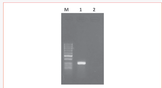
شکل ۱- تست PCR بهینه شده ژن glmM هلیکوباکتر پیلوری. M: ساین مارکر فرمنتاس ۵۰ جفت بازی، ۱: محصول ۲۹۴ جفت بازی ژن glmM هلیکوباکتر پیلوری، ۲: کنترل منفی
