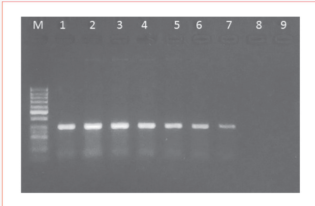
شکل ۲- تست حساسیت PCR با استفاده از رقت های متوالی DNA هلیکوباکتر پیلوری، M: ساین مارکر جفت بازی ۵۰ فرمنتاس، ۱: کنترل مثبت ۲: ۱۰۰۰۰۰۰ عدد DNA 3: 100000 عدد DNA 4: 10000 عدد DNA 5: 1000 عدد DNA 6: 100 عدد DNA 7: 10 عدد DNA 8: 1 عدد DNA 9: کنترل منفی
