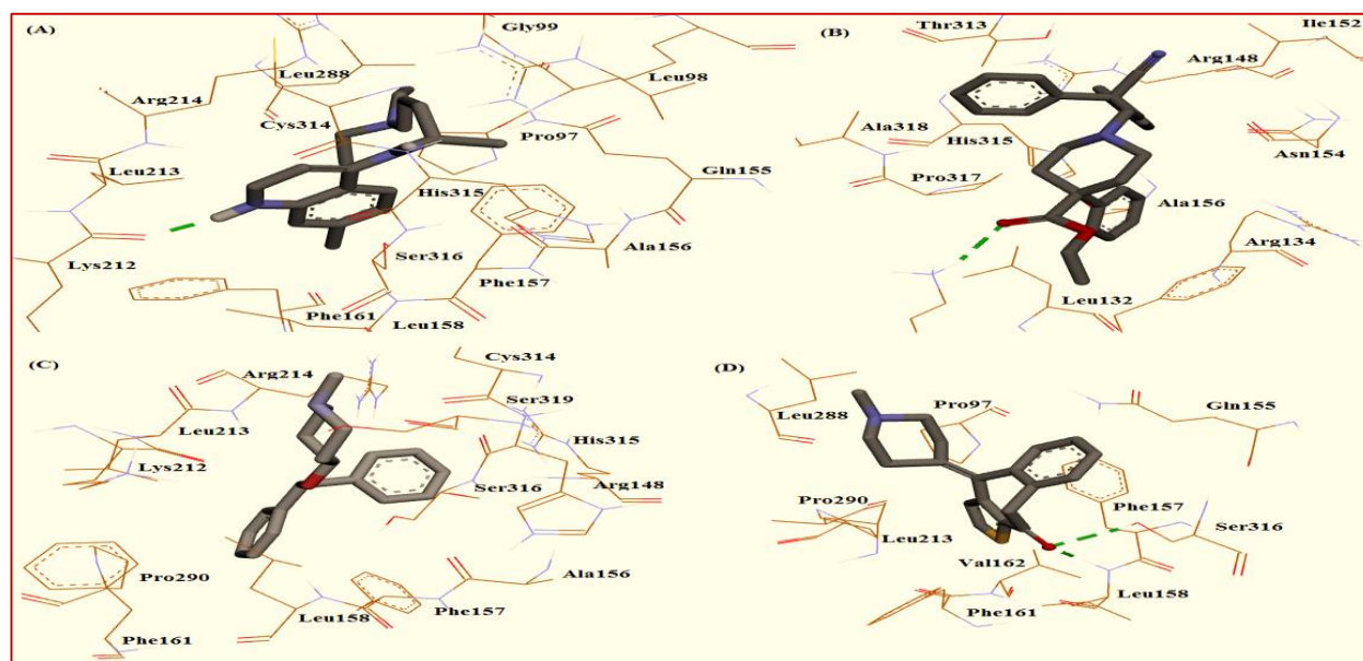
شکل ۲- بررسی اسیدهای آمینه درگیر در تشکیل پیوند هیدروفوبی و هیدروژنی (پیوندهای هیدروژنی با خط‌چین سبز نشان داده شده‌اند) با داروهای کلروکینون (A)، دی فنوکسیلات (B)، دی فنیل پیرالین (C) و کتوتیفن (D) در جایگاه اتصال گیرنده VP40
