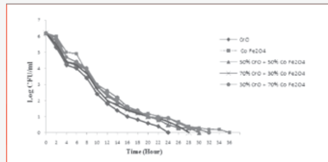
شکل ۳: محاسبه سنتیک کشندگی ۱٪ از نانوذرات CrO و \text{CoFe}_2\text{O}_4 بر روی باکتری استافیلوکوکوس اورئوس.
