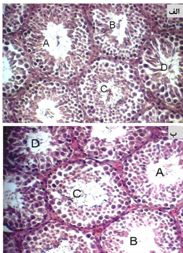
شکل ۱- مشاهده اثر رتینوئیک اسید بر فازهای اپی تلیوم منی ساز بیضه موش. الف: گروه کنترل، ب: گروه تجربی (بزرگنمایی \times 400 میکروسکوپ نوری، رنگ آمیزی H&E). A: مراحل I-II-III B: مراحل IV-V-VI-VII C: مراحل VIII-IX D: مراحل X-XI-XII
