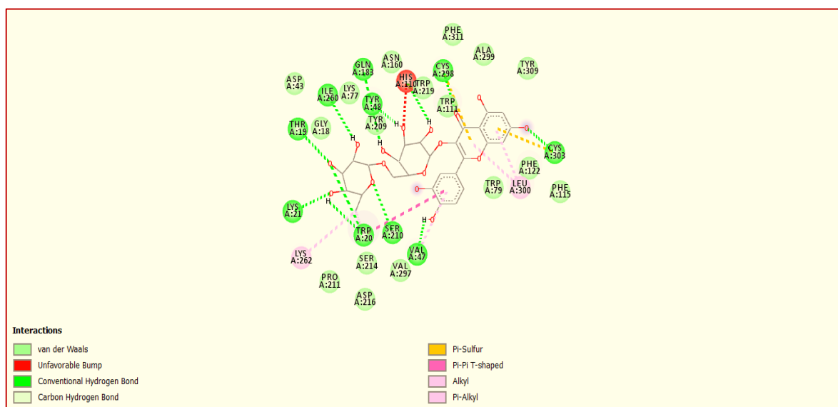
شکل ۴. برهم‌کنش‌های دوبعدی ترکیب Rutin با آنزیم آلدوز ردوکتاز (PDB ID: 1US0)
