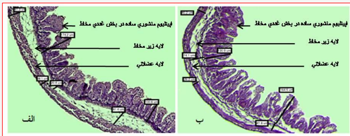
شکل ۲: تصاویر بافتی بخش غده‌ای معده شامل لایه‌های مخاط، زیر مخاط و عضلانی معده جنین ۲۰ روزه (الف) گروه شاهد و (ب) گروه تجربی دوز ۳۰۰ mg/kg آسپرین. (بزرگنمایی ۱۰۰× و رنگ آمیزی هماتوکسیلین-ئوزین).
