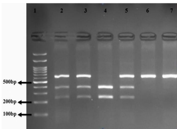
شکل ۲- نتایج RFLP بر روی ژل آگارز. ستون ۱: ladder 100bp، ستون ۲، ۳ و ۴: هتروزیگوت G/A، ستون ۵ و ۶: هموزیگوت A/A، ستون ۷: هموزیگوت G/G
